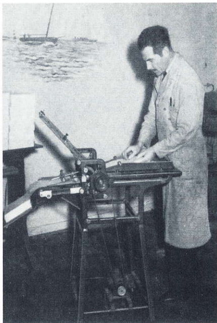
Koos Klaton achter de vouwmachine. Deze machine vouwde de gedrukte vellen met een snelheid van plm. 3000 ex per uur.
